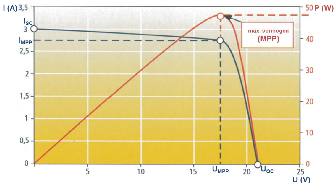
Figuur 40: I-U en P-U curve van een module – bron: [8]
