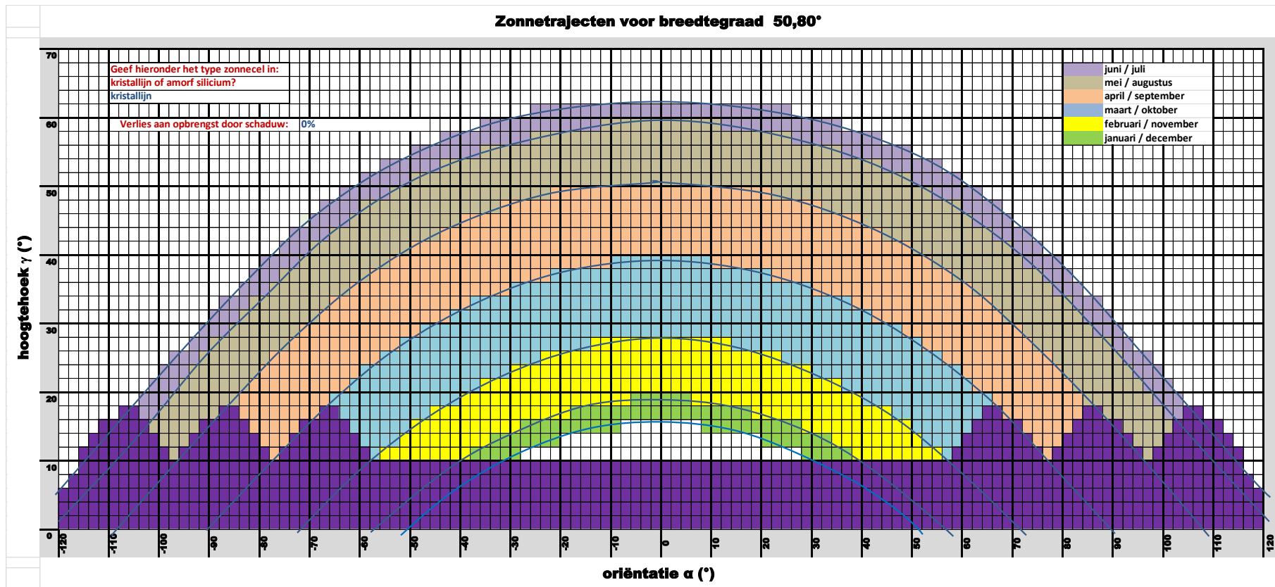
Figuur 71: zonnetrajecten overgebracht naar een Excel rekenblad
