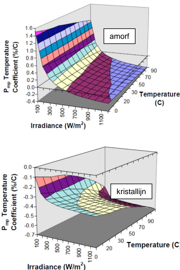
Figuur 43: temperatuurcoëfficiënt in functie van de instraling en temperatuur voor twee verschillende PV-modules: bovenaan amorf Si (UPM-880 tandem module van USSC) onderaan kristallijn Si (ASE-300-DG/50 module van ASE Americas) bron: [9]
