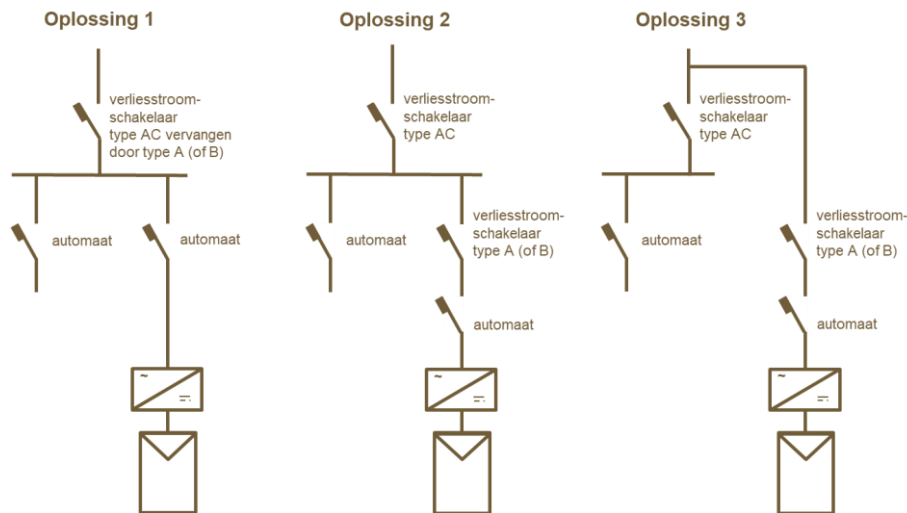
Figuur 28: installatie met verliesstroomschakelaar van type AC: verplichte verliesstroomschakelaar van type A bij uitbreiding met een PV-installatie
