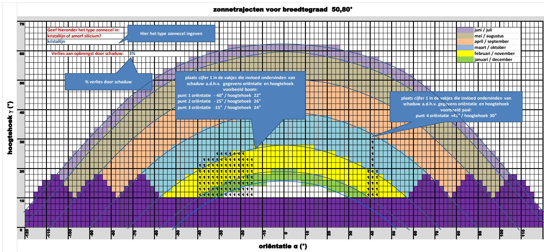
Figuur 72: voorbeeld van een ingevuld "Schaduw rekenblad"
