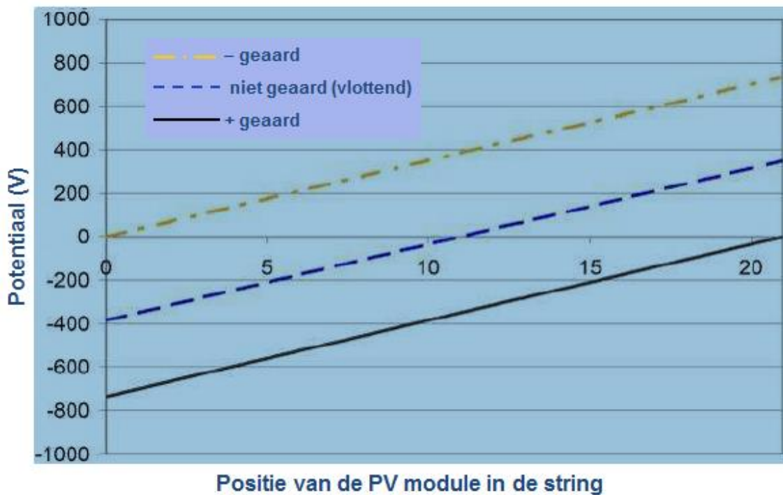
Figuur 44: aardingsschema's voor een PV-installatie van 750 V Bron: [10]
