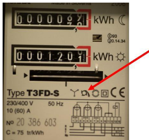
Figuur 5: symbool voor een teruglooprem op een Ferrarimeter
