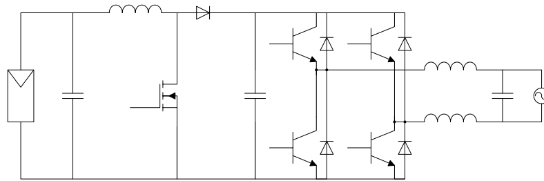
Figuur 58: voorbeeld van een transformatorloze omvormer
