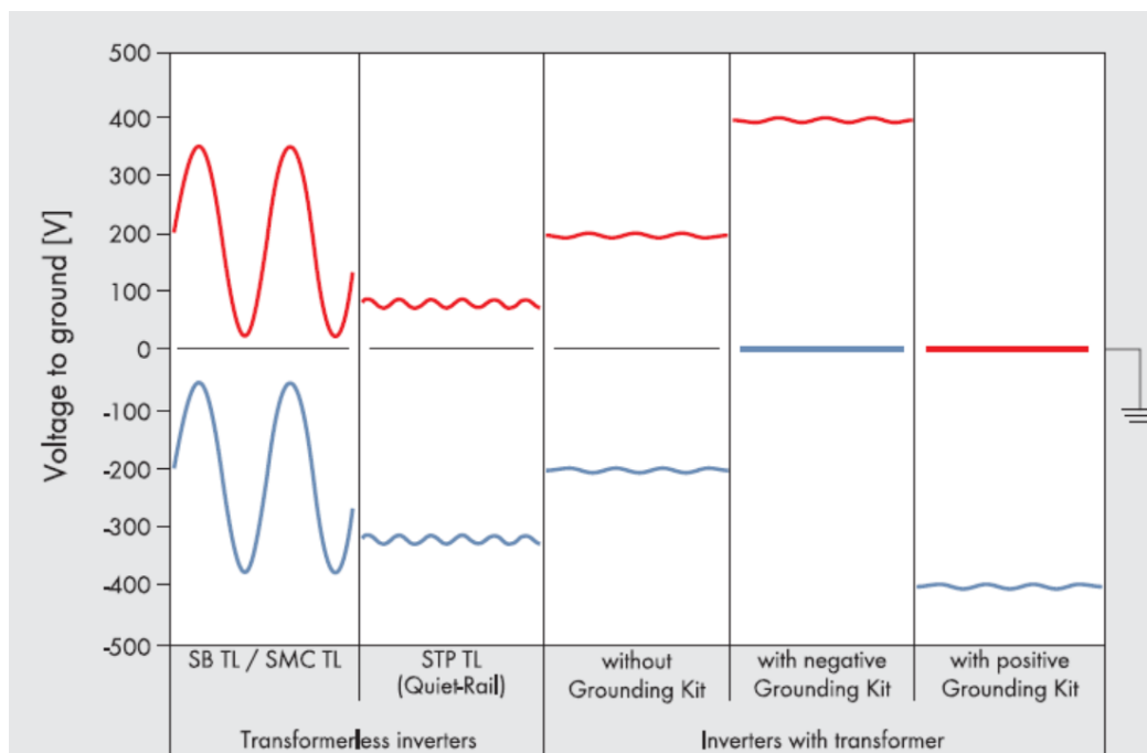
Figuur 60: potentiaal van de + t.o.v. de aarde en van de – t.o.v. de aarde (hier bij 400 V DC) in functie van de omvormertechnologie Bron: SMA
