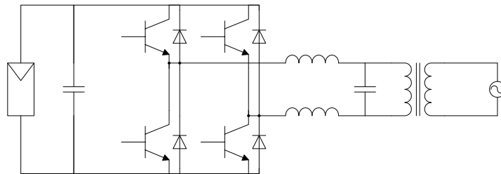
Figuur 56: voorbeeld van een omvormer met lijnfrequentietransformator
