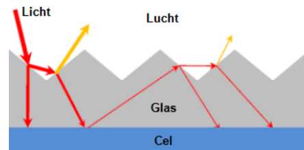
Figuur 39: gedrag van invallend licht bij gestructureerd glas – bron: [6]
