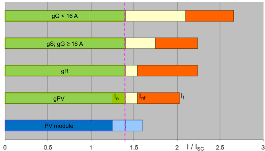
Figuur 63: werkingsgebied van verschillende types smeltveiligheid met I_n = 1,4 \times I_{sc \text{ stc}}
