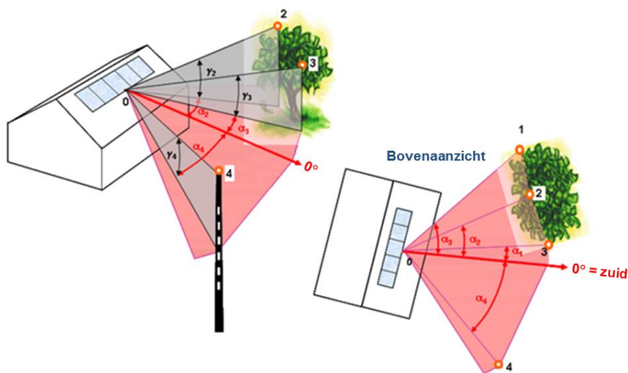
Figuur 68: kaart van voorwerpen die schaduw werpen op een PV-installatie
