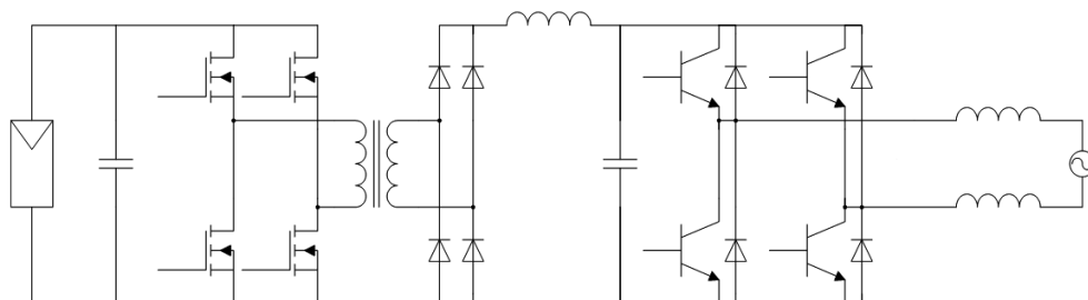
Figuur 57: voorbeeld van een omvormer met hoogfrequent-transformator
