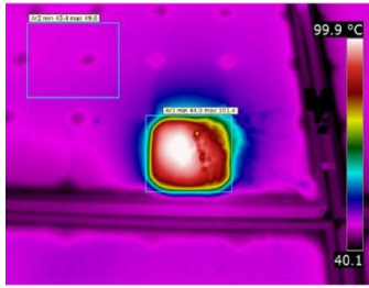
Figuur 35: hot spot in een PV-module
