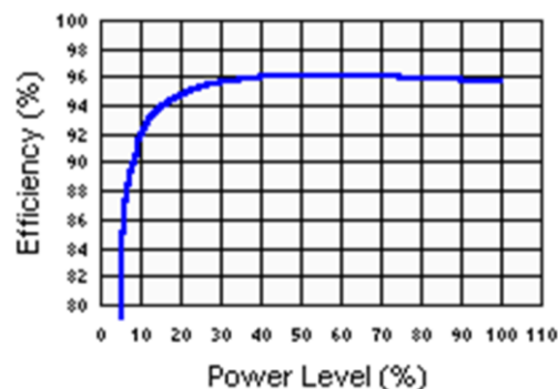
Figuur 53: voorbeeld van het omzettingsrendement van DC naar AC in een omvormer, in functie van het percentage van het maximaal vermogen.
